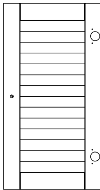
5 Left door panel (505 x 267mm)
