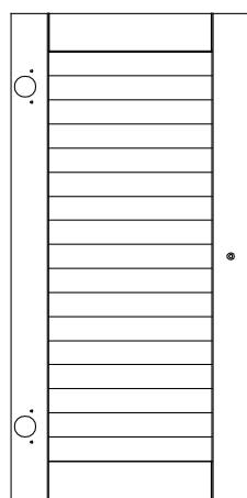
6 Right door panel (286 x 594mm)
