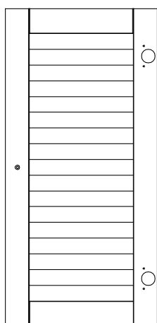
5 Left door panel (286 x 594mm)
