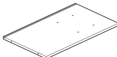
3 Bottom shelf x 1 (53.8(w) x 32(d)cm)
