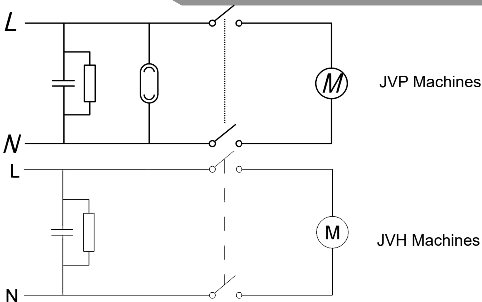
Schematic Diagram - Schaltplan - Schéma électrique - Bedradingsschema - Diagrama esquemático - Schema apparecchio - Esquema eléctrico
