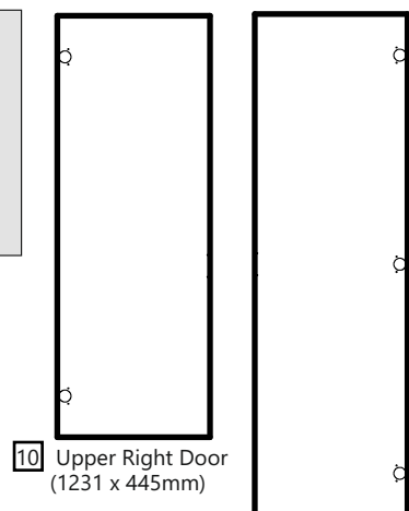
12A Left Big Door (1462 x 445mm)
