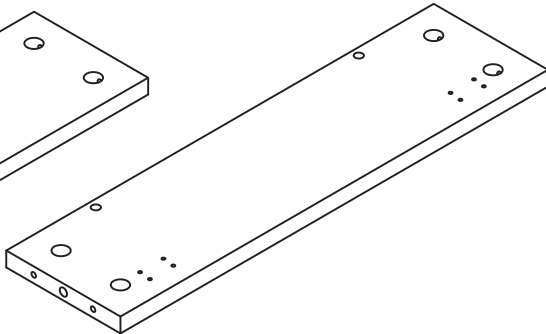
3 Right Side Panel x 1 47(w) x 12.5(d) x 1.5(h)cm
