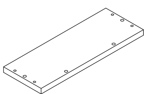
1 Top&Bottom Panel x 2 34(w) x 12.5(d) x 1.5(h)cm
