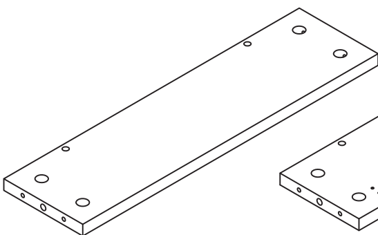
2 Left Side Panel x 1 47(w) x 12.5(d) x 1.5(h)cm
