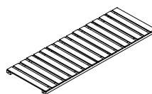
7 Bottom Rack x 1 91.3cm x 32cm x 2.5cm
