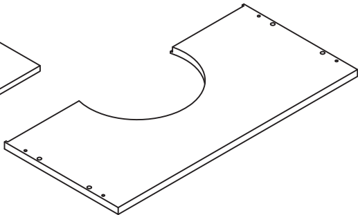
6 Bottom Panel x 1 60(w) x 28.5(d) x 1.5(h)cm
