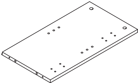
3 Right Side Panel x 1 51(w) x 28.5(d) x 1.5(h)cm
