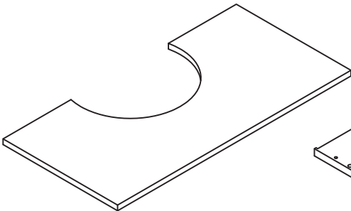
5 Shelf x 1 56.8(w) x 28(d) x 1.2(h)cm
