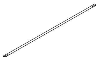
14f Slat x 14 (1217mm)
